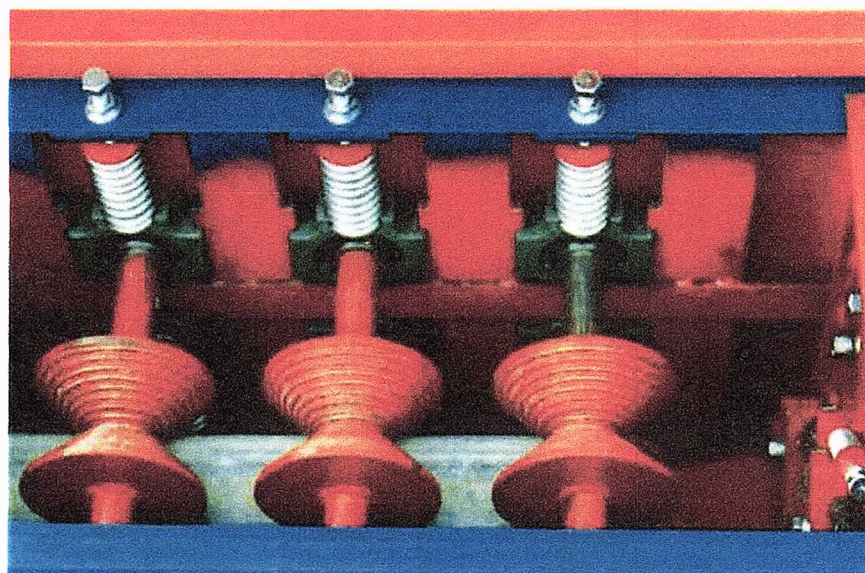
特殊クラッシャーローラと特殊ブラシボックス
